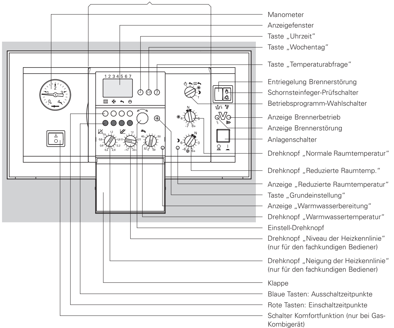
Standard-Bedieneinheit (herausnehmbar)
