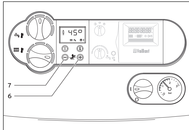
Abb. 4.16 Schornsteinfeger-Betrieb einschalten
