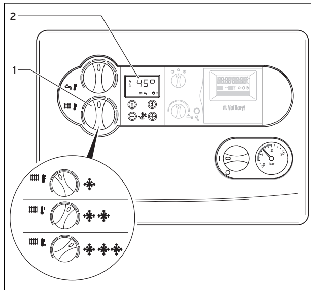
Abb. 4.8 Vorlauftemperatur-Einstellung ohne Regelgerät
