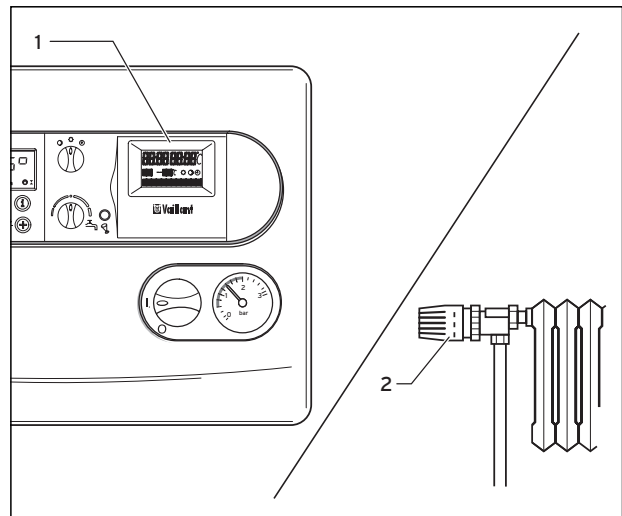
Abb. 4.10 Raumtemperaturregler/witterungsgeführte Regler einstellen
