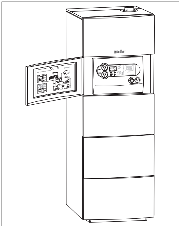
Abb. 4.1 Verkleidungstür öffnen
