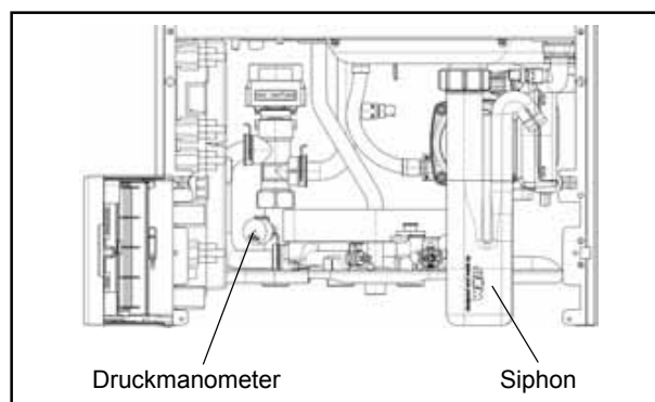
Bild: Druckmanometer und Siphon
