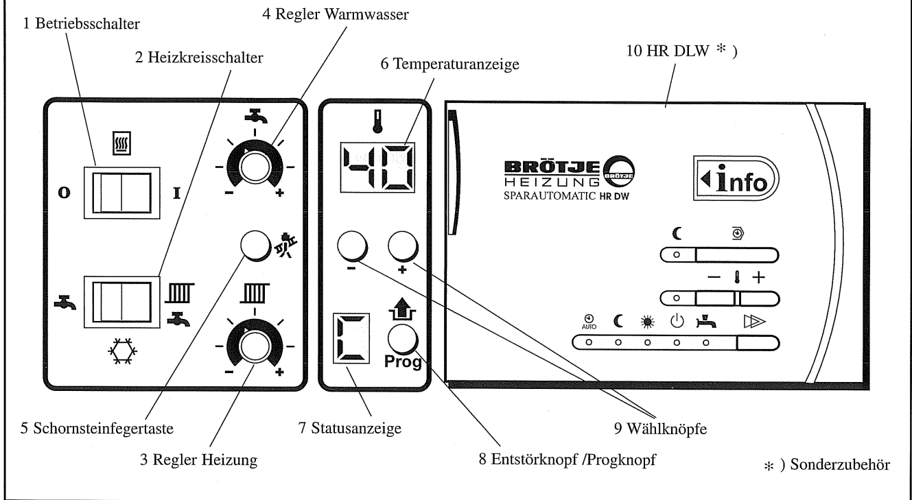
Abb. 1 Bedientafel
